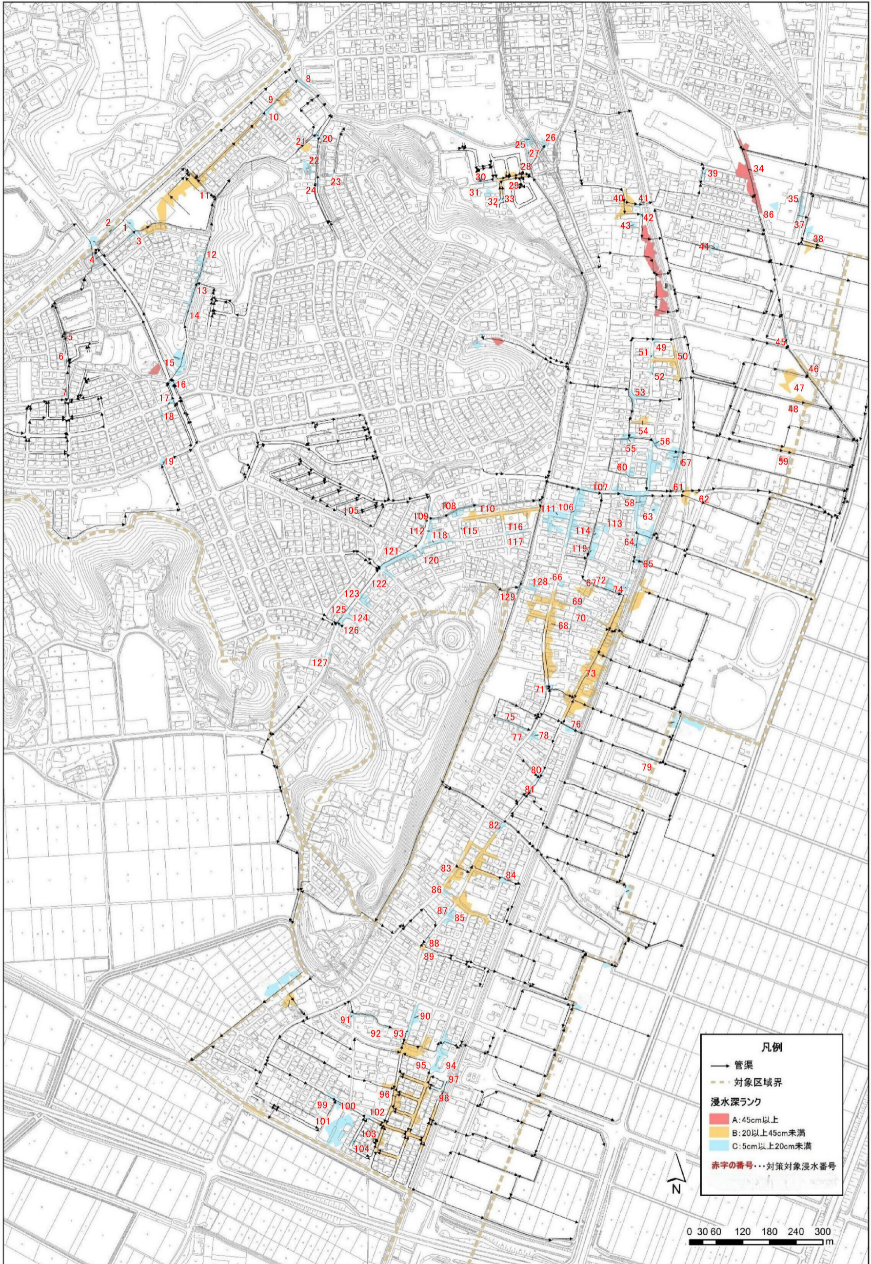
図-2 浸水箇所位置図(小規模管路対策)＜館腰地区＞
