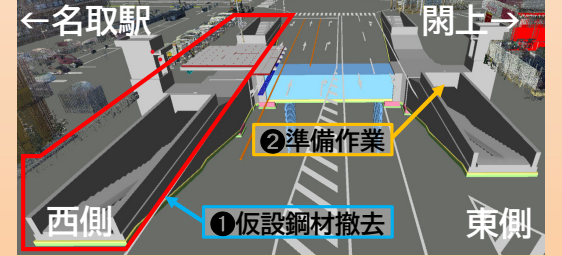
特殊材料を地中に充填しながら鋼矢板を引抜きます。
