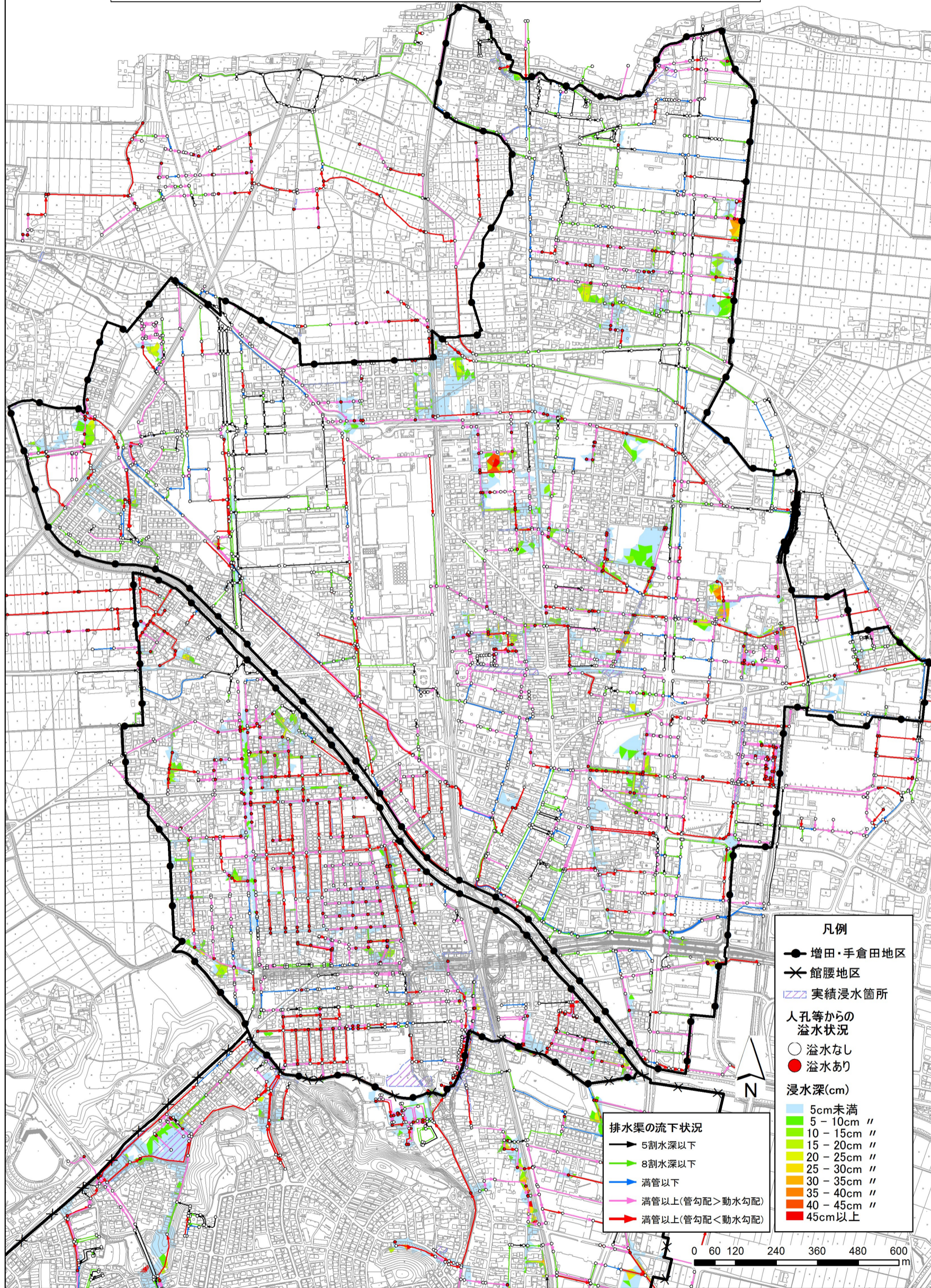
10年確率降雨[52mm/h]シミュレーション結果（増田・手倉田地区）
