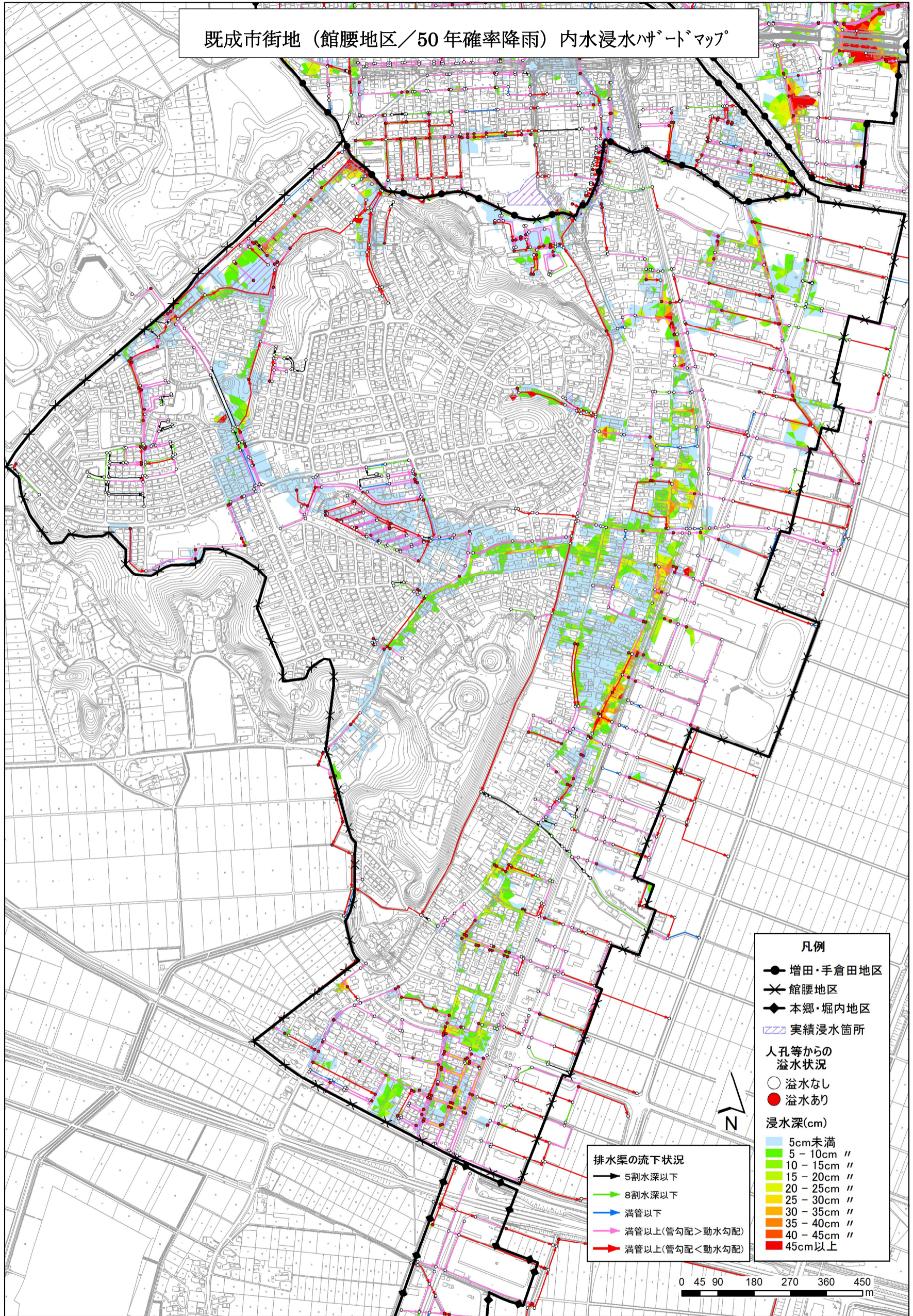
50年確率降雨[74mm/h]シミュレーション結果（館腰地区）
