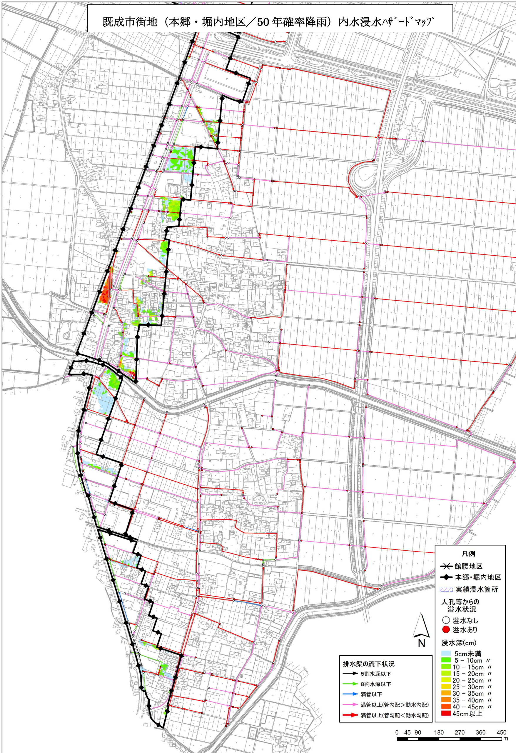
50年確率降雨[74mm/h] シミュレーション結果 (本郷・堀内地区)
